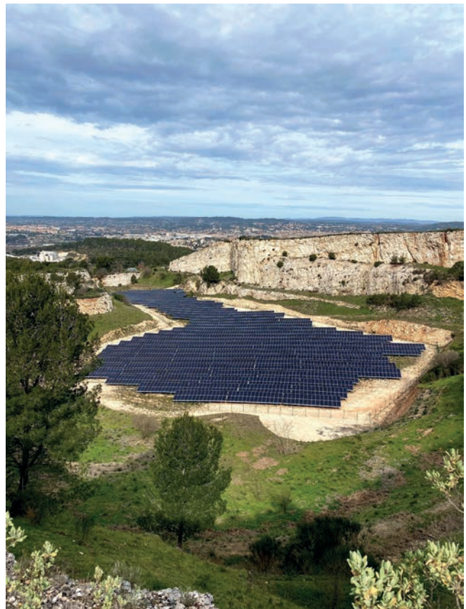
La centrale solaire des Brègues d'Or, avec l'Hôpital privé de Provence en contrebas.
